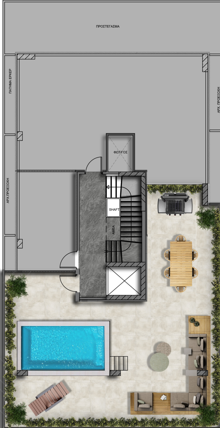
ΚΑΤΟΨΗ ΔΩΜΑΤΟΣ
