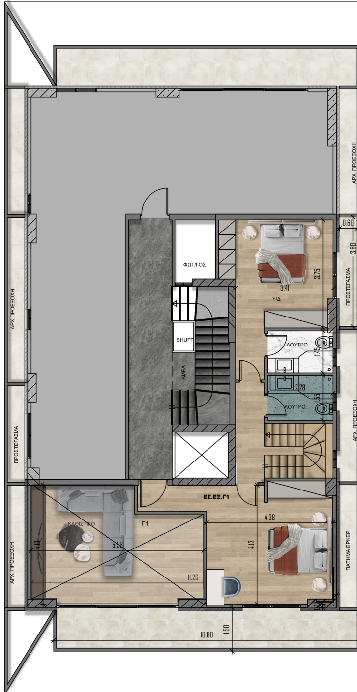
ΚΑΤΟΨΗ ΕΣΩΤ. ΕΞΩΣΤΗ Γ' ΟΡΟΦΟΥ
